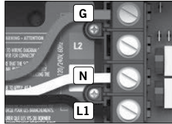
120 V (*3 wires)
