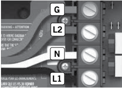
240 V (4 wires)
