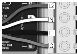
240 V (4 wires)
